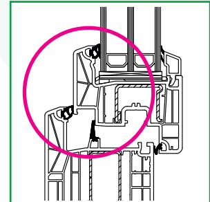
Optionale Mitteldichtung
