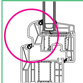
Rundflügel (halbflächenversetzt)
