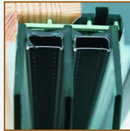
3-fach-Verglasung mit "warmer Kante" im Standard
