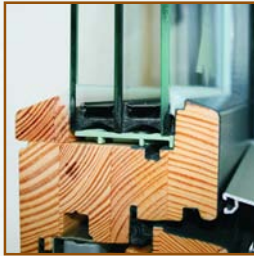
bis zu 50 mm Glasstärke
